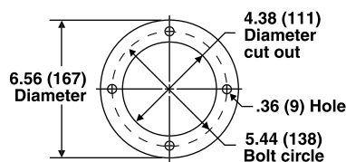
VERSA FLANGE BOLT CIRCLE
